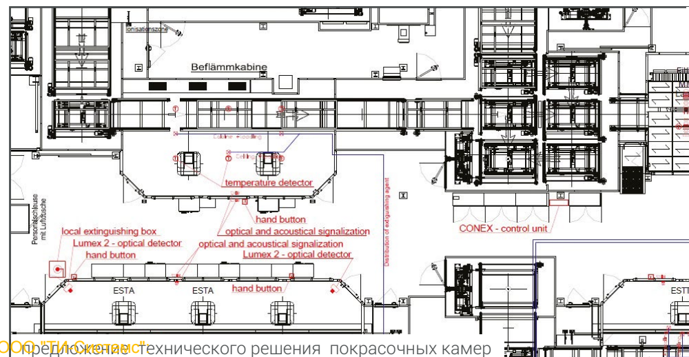
камера распыления для нанесения органических жидких окрасочных материалов
